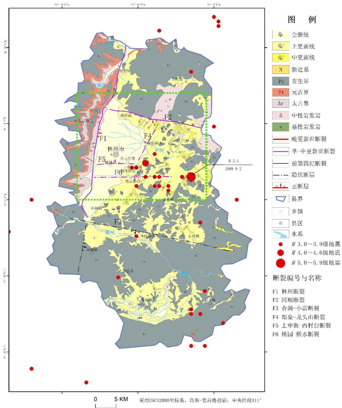
林州市1: 250000地震构造图
