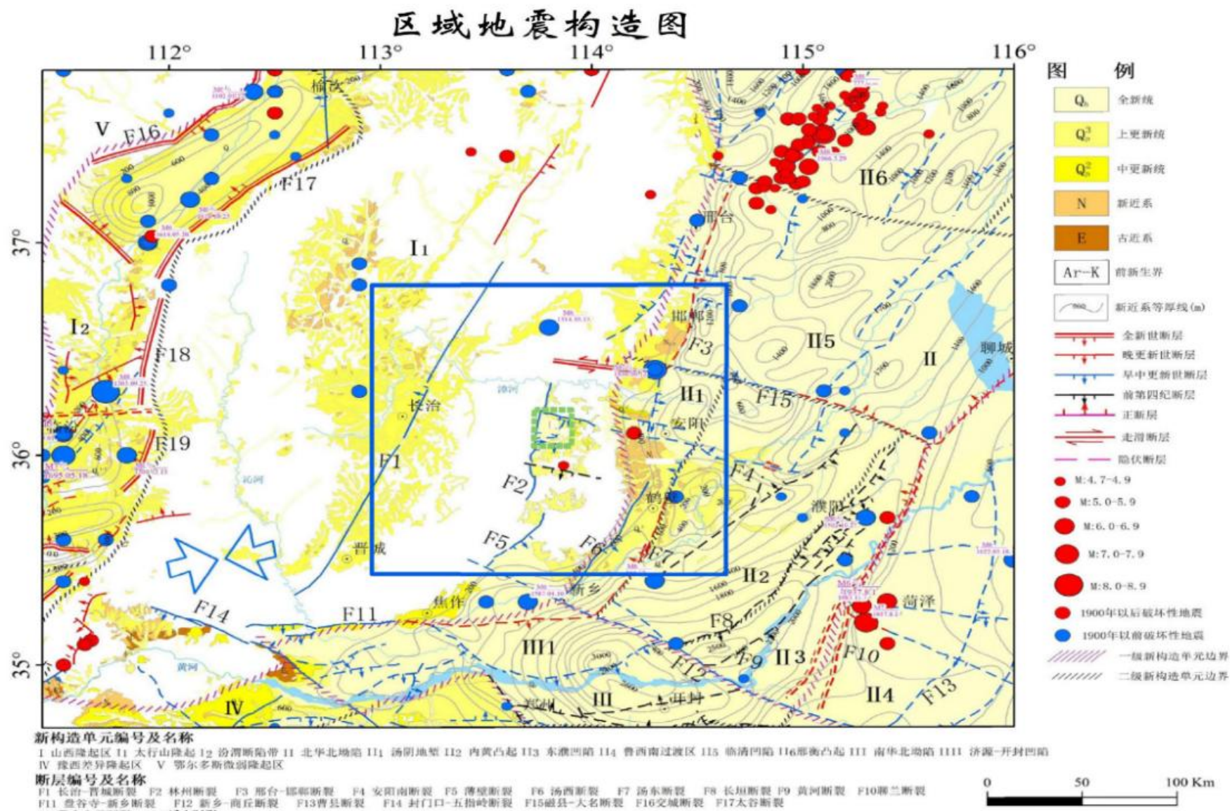
图 2.3-3 探测区及邻区地震构造图（绿色线为目标区范围、蓝色线为探测区范围）
