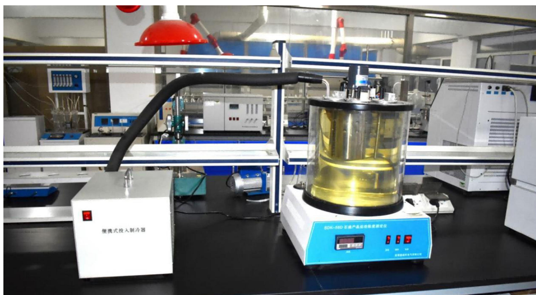
石油产品运动粘度测定仪
