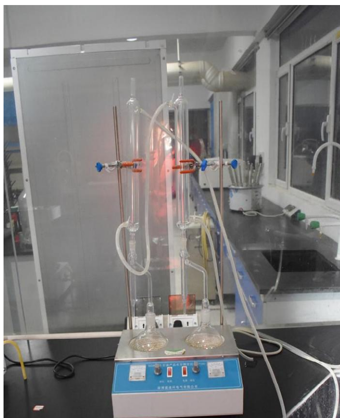
石油产品水分测定仪
