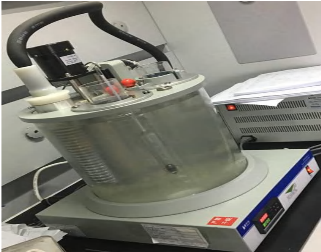
石油产品色度试验器
